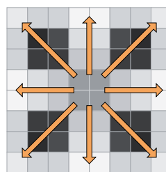
双三次插值算法
