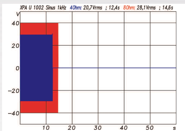
ABB. 13: Verhalten der XPA U 1002 bei einem konstant anliegenden Sinussignal für maximale Ausgangsleistung an 2 \times 4 \Omega (bl) und an 2 \times 8 \Omega (rt)
