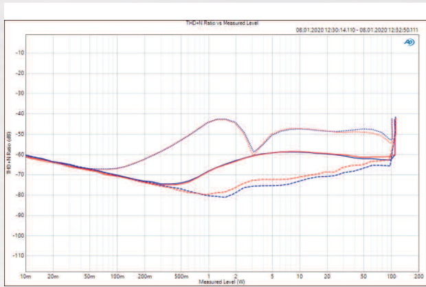
ABB. 07: Verzerrungswerte (THD+N) für Kanal 1 (bl) und 2 (rt) in Abhängigkeit von der Leistung (x-Achse) für eine Last von 2 \times 4 \Omega gemessen bei 100 Hz (gestrichelt), bei 1 kHz (durchgezogen) und 6,3 kHz (gepunktet)
