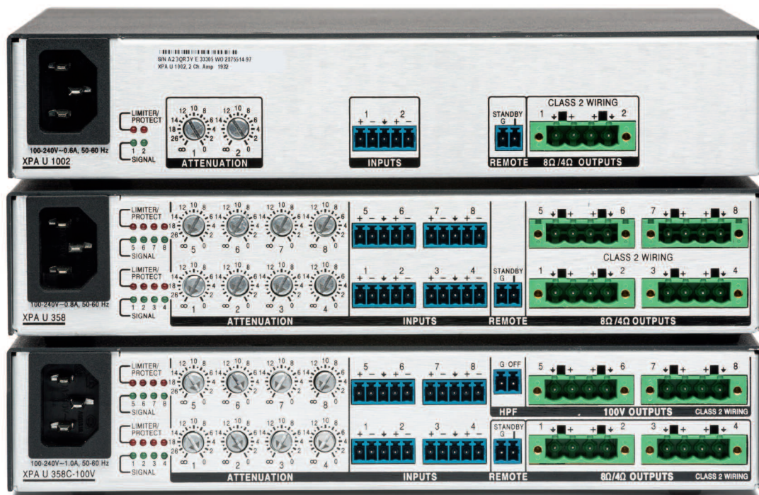
BILD 03: Die drei Modelle von der interessanteren Rückseite mit Ein- und Ausgängen auf Klemmleisten, Gain-Trimmern für alle Kanäle und Signal Present sowie Limiter/Protect LEDs auch auf der Rückseite!
