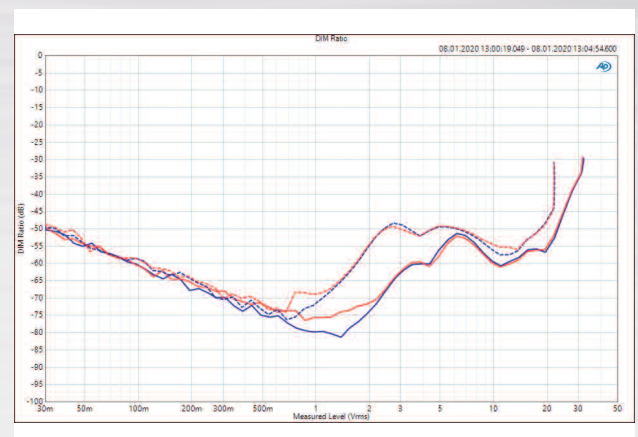
ABB. 10: Transiente Intermodulationsverzerrungen (DIM) für Kanal 1 (bl) und 2 (rt) in Abhängigkeit von der Ausgangsspannung (x-Achse) für eine Last von 2 \times 4 \Omega (durchgezogene Linien) und 2 \times 8 \Omega (gestrichelte Linien)
