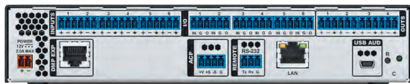
DMP 64 Plus C - 后面板
