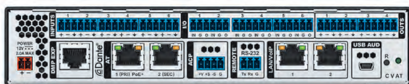
DMP 64 Plus C V AT - 后面板
