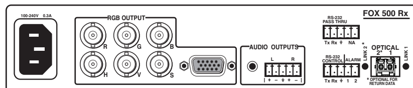
FOX 500 Rx - 背面
