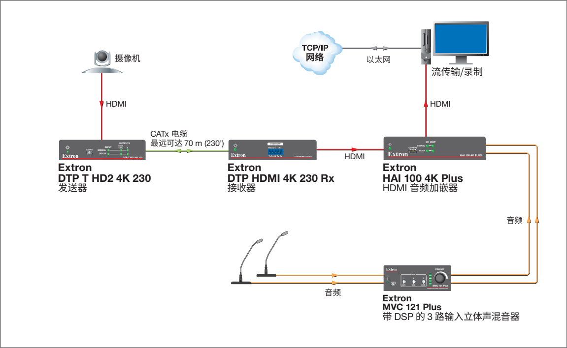
HAI 100 4K Plus 应用于流媒体传输工作站
