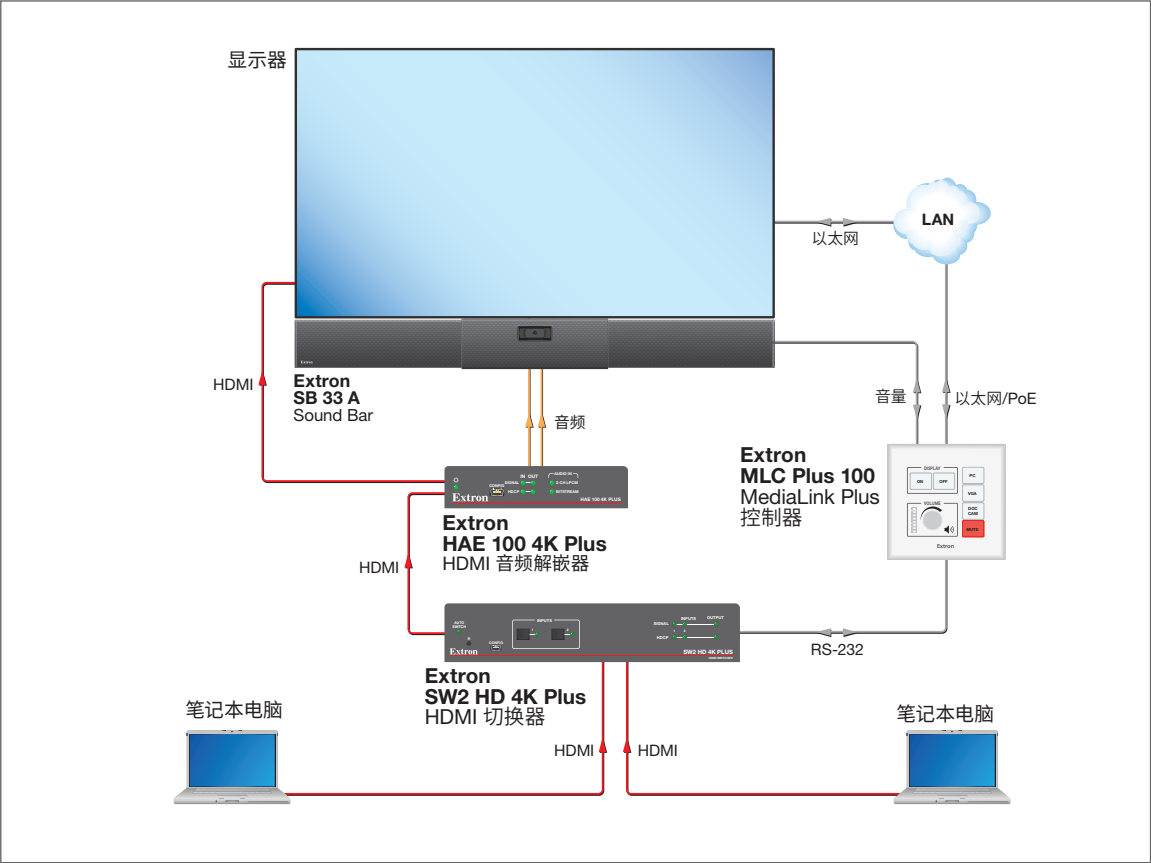
HAE 100 4K Plus 和 SB 33 A Sound Bar 应用于紧凑型会议室
