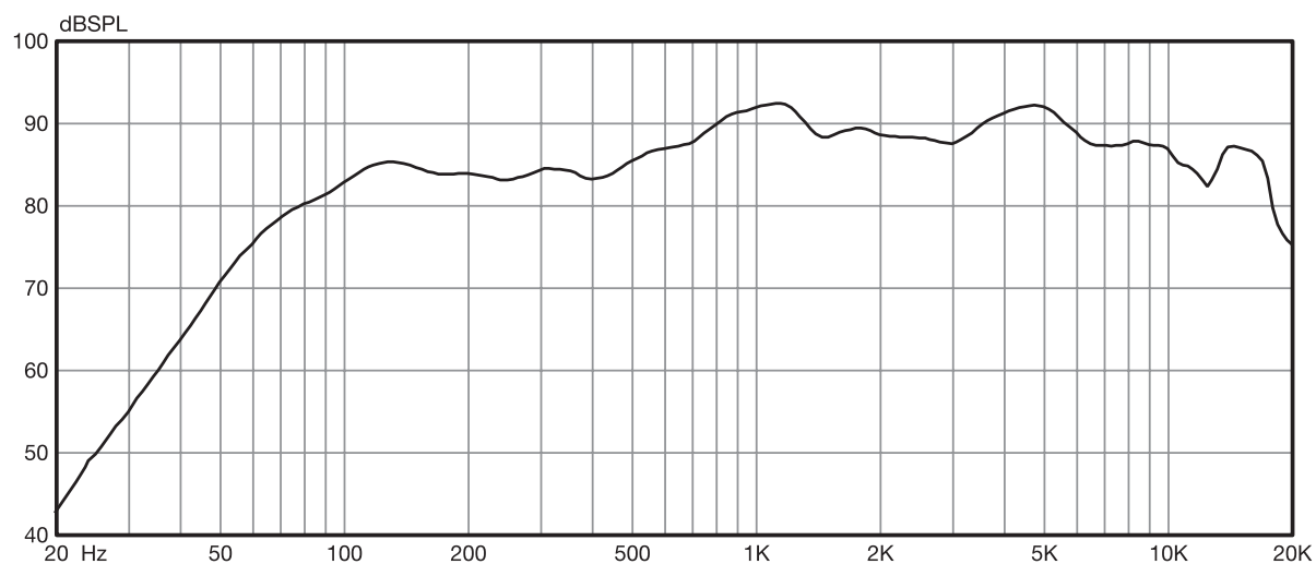
声压级 vs. 频率 - 1W / 1 m 响应, 全空间 ( 4\pi )
