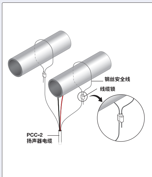
图 1: 可使用随附的 PCC-2 扬声器电缆将 SF 26PT 悬挂在天花板下方
