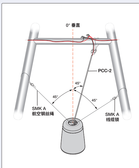
图 4: 可选的 SMK A 钢丝绳套件安装示例
