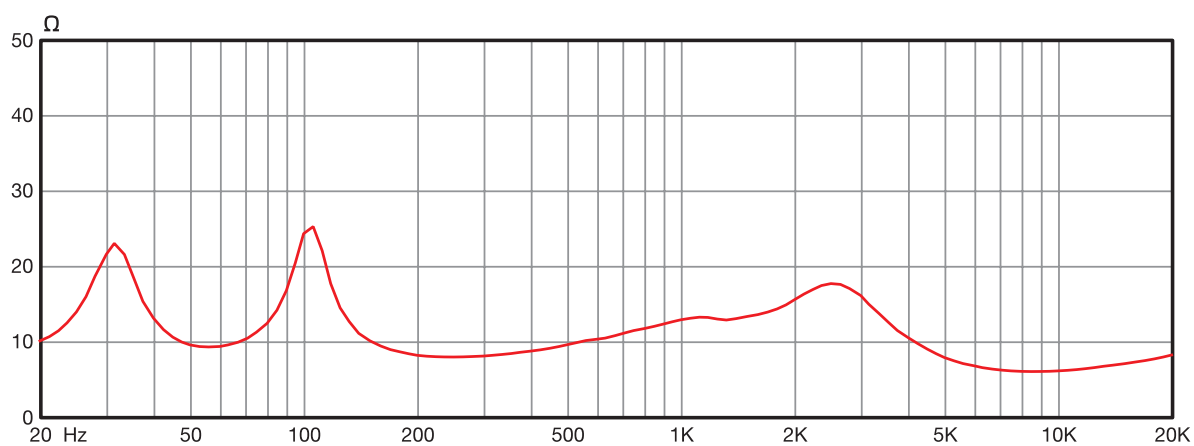
阻抗 vs. 频率
