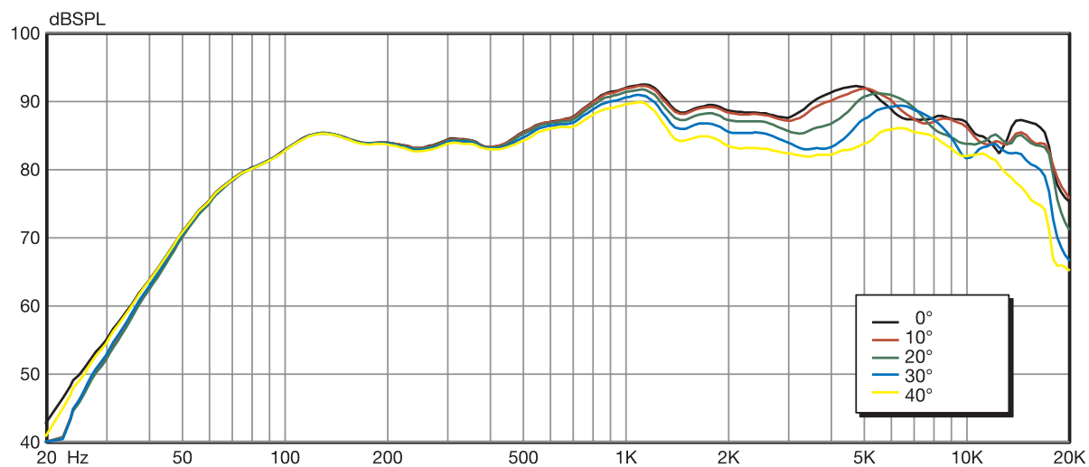
声压级 vs. 频率 - 水平离轴响应, 全空间 ( 4\pi )
