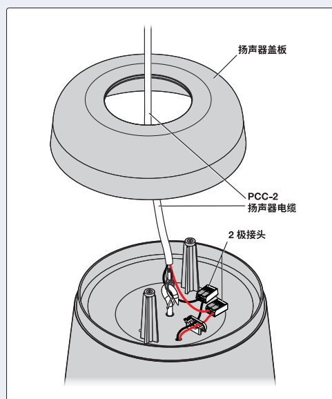
图 2: PCC-2 扬声器电缆的另一端连接至 SF 26PT 顶部
