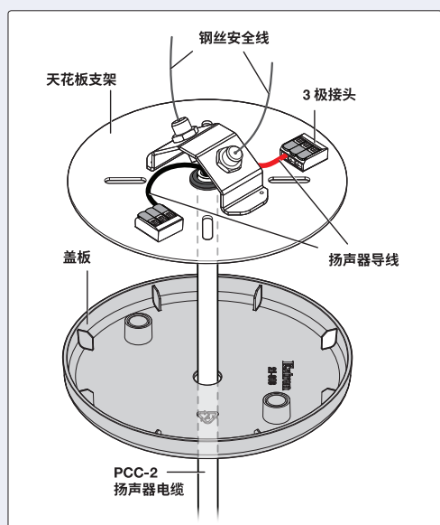
图 3: 可选 SMK C SF 26PT 天花板表面安装套件详情图
