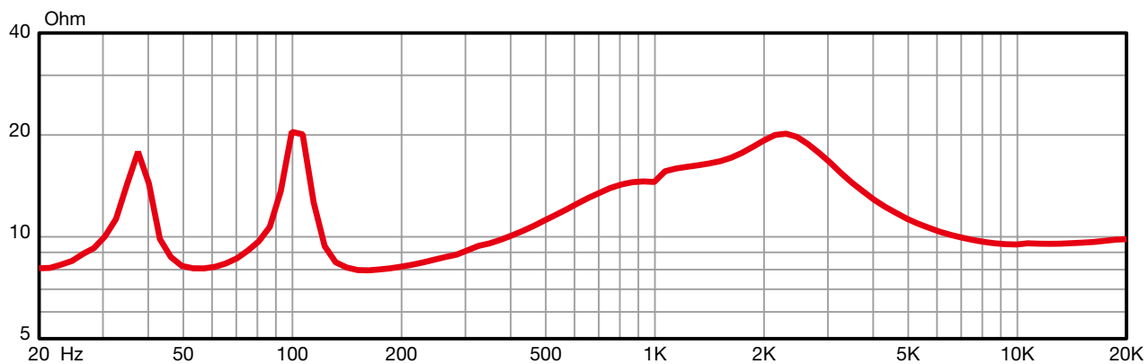
阻抗与频率
