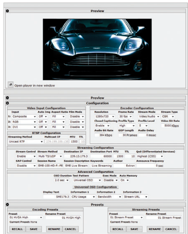
SME 100 编码配置
