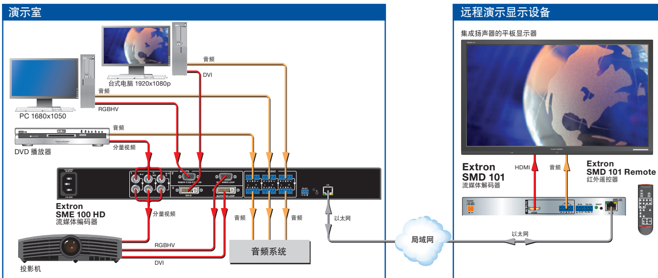
从 SME 100 到 SMD 101 解码器的流媒体演示线路图
