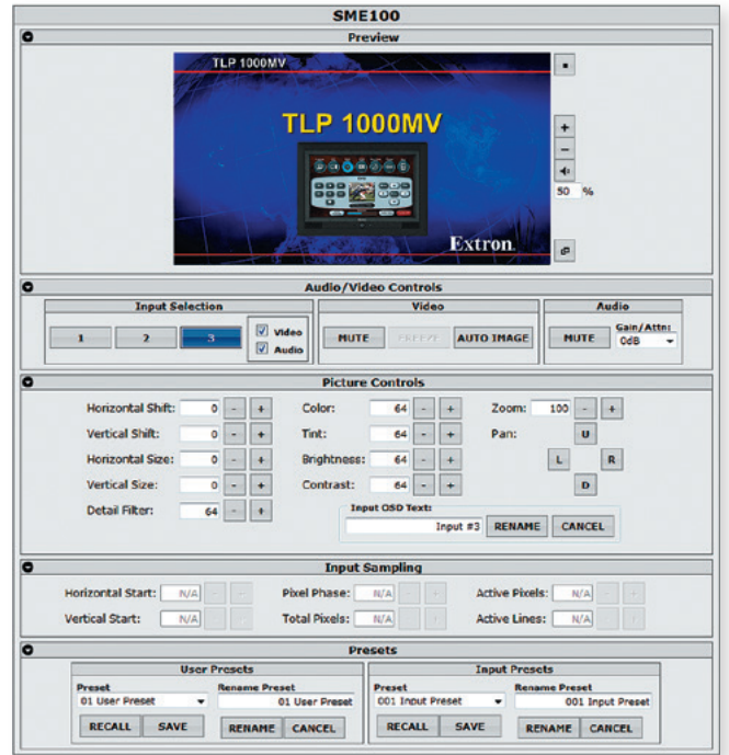
SME 100 信号输入控制
