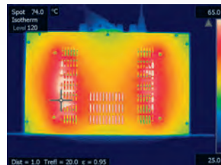
红外温度记录器显示了 AB 类和 XTRA 系列 D 类放大器的热量输出对比
